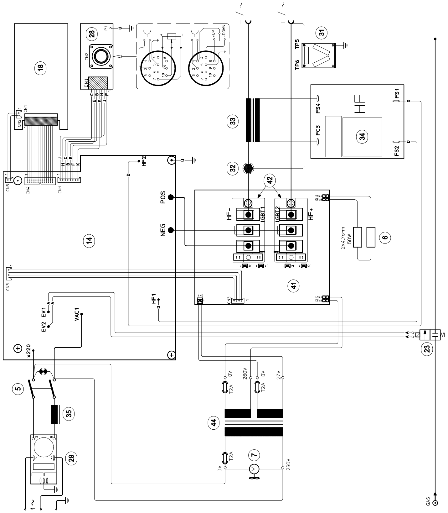
Art. 115: SCHEMA ELETRICO - WIRING DIAGRAM - ELEKTRISCHER SCHALTPLAN - SCHEMA ELECTRIQUE - ESQUEMA ELECTRICO
