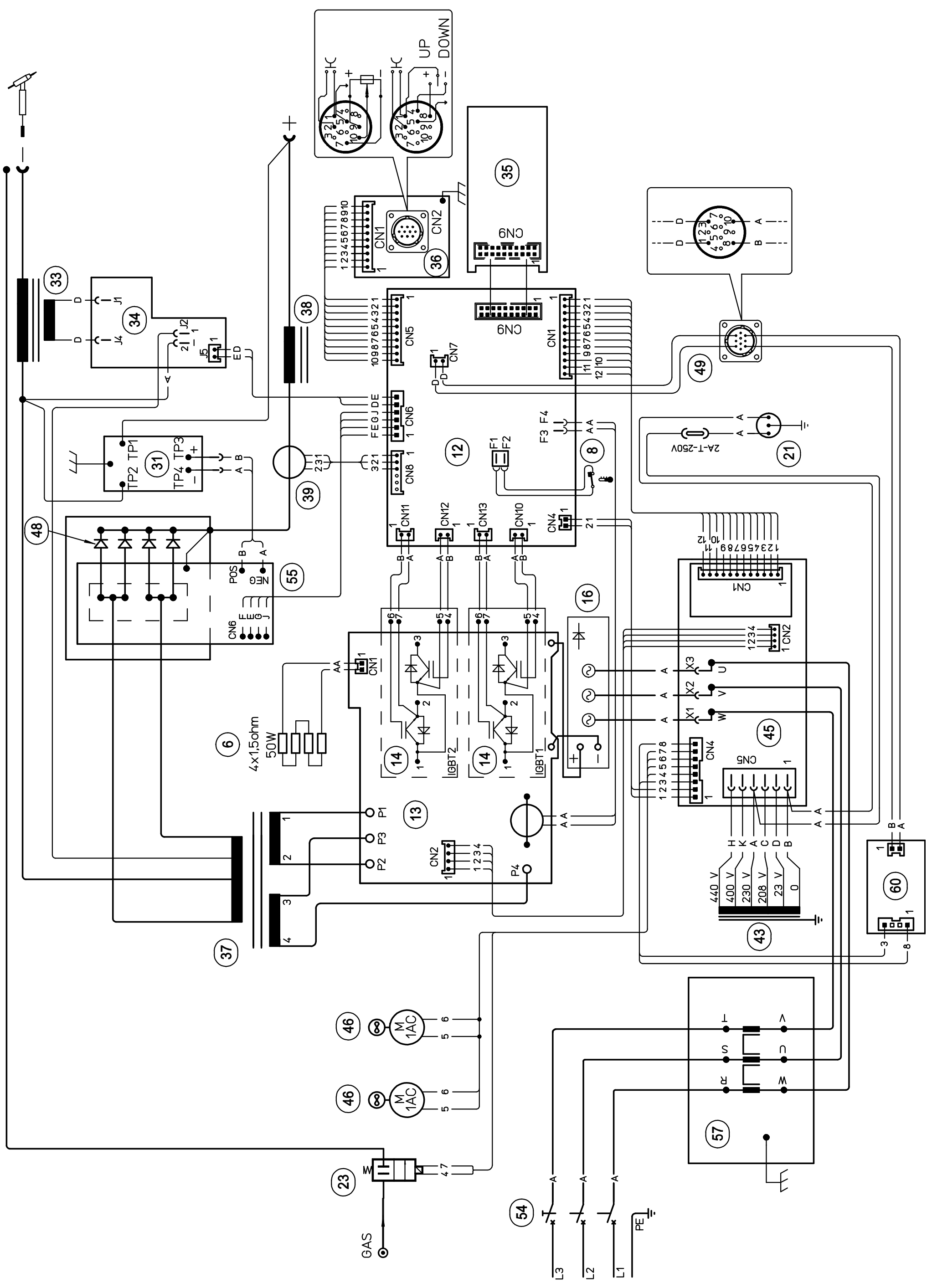
Art. 120: SCHEMA ELETTICO - WIRING DIAGRAM - ELEKTRISCHER SCHALTPLAN - SCHEMA ELECTRIQUE - ESQUEMA ELECTRICO
