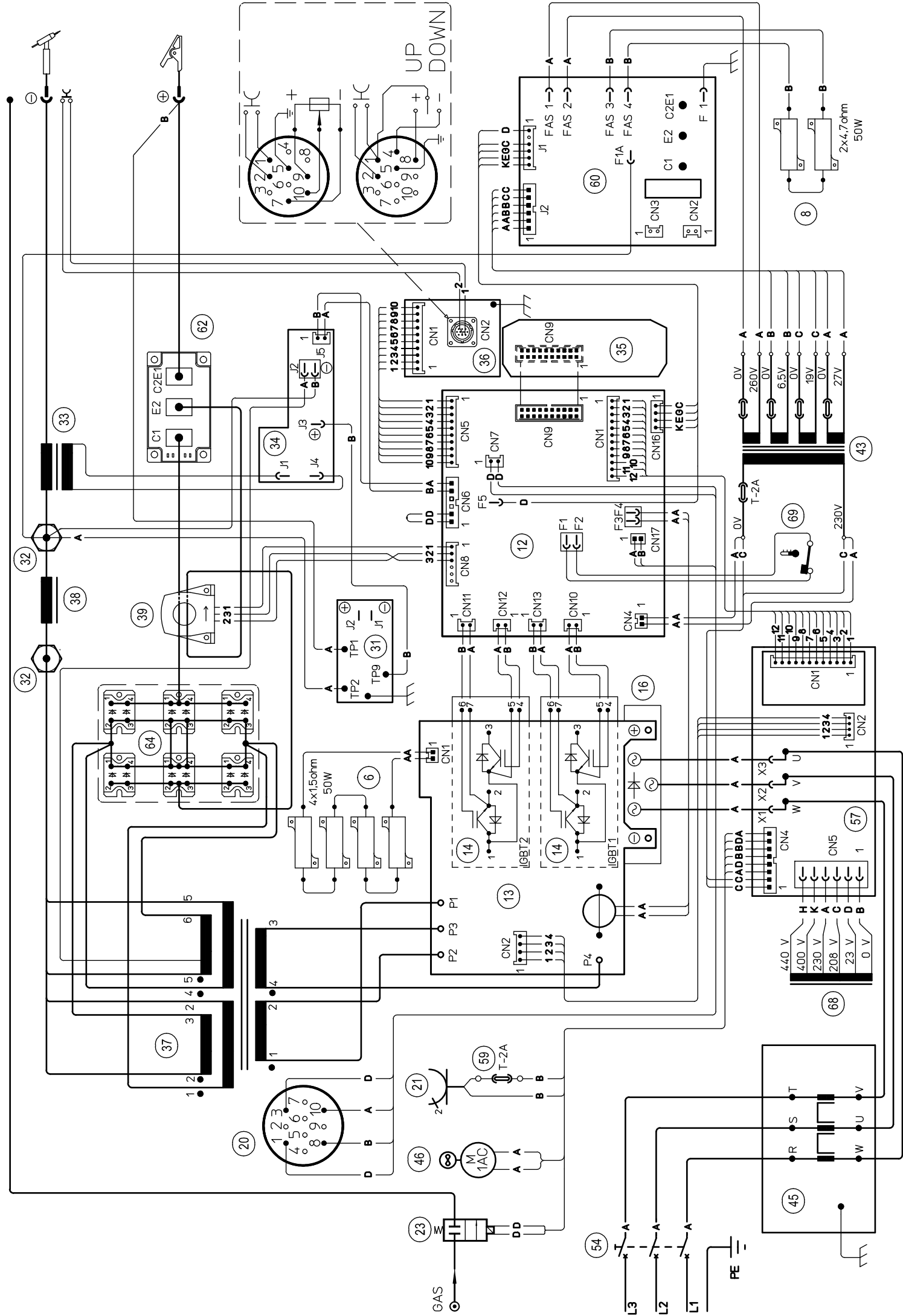
Art. 128: SCHEMA ELETTICO - WIRING DIAGRAM - ELEKTRISCHER SCHALTPLAN - SCHEMA ELECTRIQUE - ESQUEMA ELECTRICO
